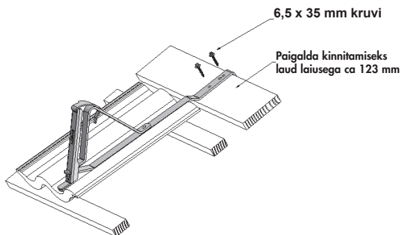
Joonis 11. Lisaroovitise paigaldus lumetõkke- ja käigusilla kanduritele.
