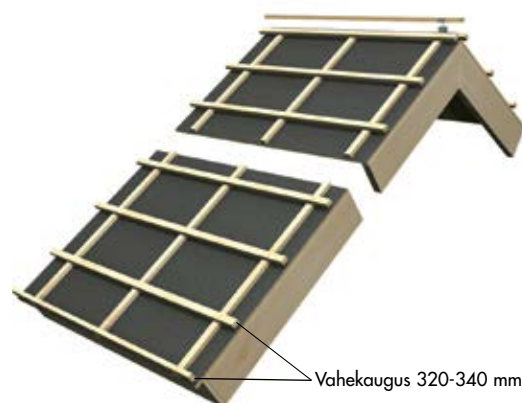
Pilt 4. Katuse alusroovitise paigutus.
