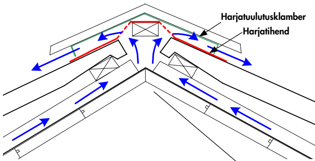
Joonis 12: Harja lahendus harjakivi ja harjatuulutusklambriga.
